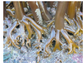
Іл. 26. Ризоїди бурих водоростей
