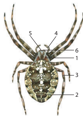
Іл. 110. Зовнішня будова павука-хрестовика:
