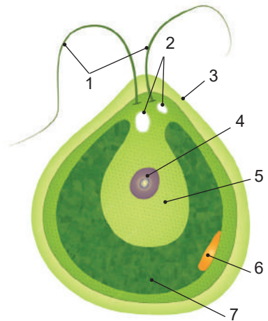
Іл. 19. Будова хламідомонади:
