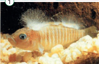
Іл. 69. Несправжні гриби: 1 – сапролегнія паразитарна; 2 – плазмопара виноградна; 3 – фітофтора інфекційна
