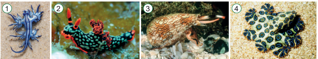
Іл. 94. Отруйні молюски: 1 – главк атлантичний; 2 – немброта сутінкова; 3 – конус географічний; 4 – блакитнокільчастий восьминіг
