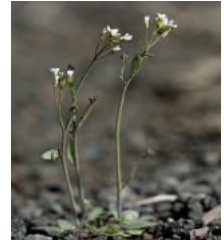
Іл. 58. Гусимка звичайна – відомий модельний організм
