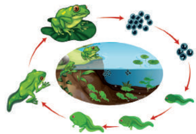
Іл. 138. Розвиток жаби (ікра – пуголовка – доросла стадія)
