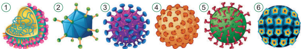
Іл. 5. Віруси-збудники захворювань людини: 1 – вірус грипу; 2 – аденовірус С (ГРВІ); 3 – вірус імунодефіциту людини (СНІД); 4 – вірус гепатиту В; 5 – рота-вірус (кишкові інфекції); 6 – папіломавірус (бородавки та новоутворення)
