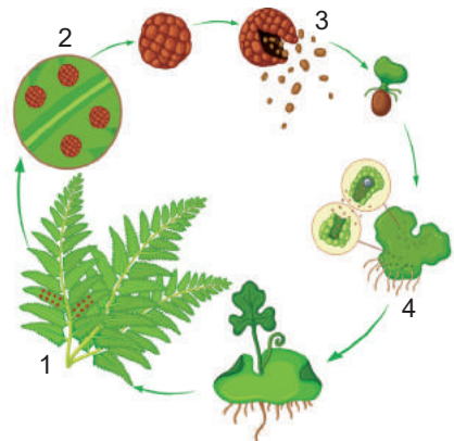
Іл. 42. Цикл відтворення папороті: 1 – спорофіт; 2 – соруси; 3 – спори; 4 – гаметофіт
